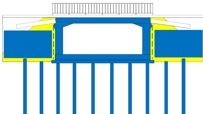
kontur obejmujący rozmieszczenie kolumn żwirowych
